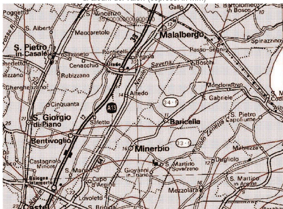
Figura 4.3 – Isolinee della precipitazione estrema cumulata (durata 6 h) per l'area di interesse, con indicazione di alcuni dei valori (espressi in mm)
