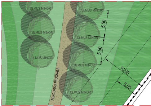
PARTICOLARE 1 - SCALA 1:250
